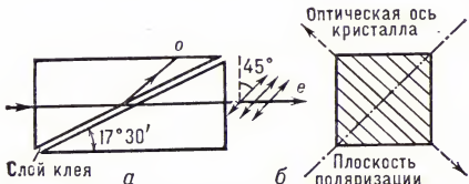
Рис. 7. Поляризационная призма Франка — Риттера (клей — канадский бальзам): а — вид сбоку; б — вид по ходу луча. Оптические оси кристаллических прямоугольных призм направлены под углом 45^\circ к плоскости рисунка а и под углом 90^\circ к плоскости колебаний электрического вектора необыкновенного луча (его плоскости поляризации).
